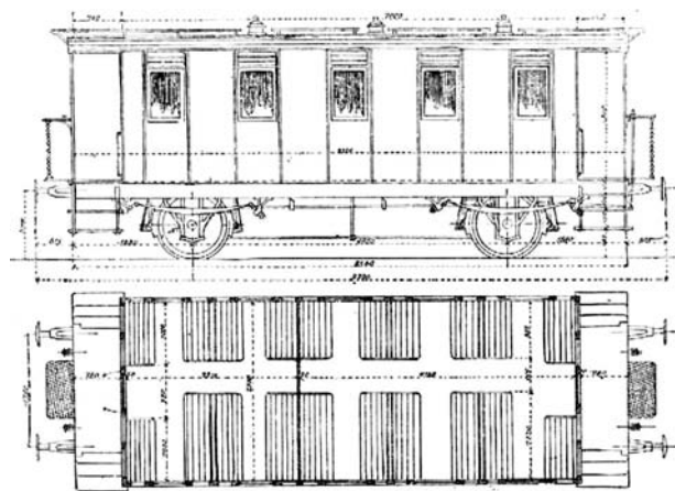
A Déli Vasút két (az egyik I. és II. osztályú, a másik III. osztályú) személyszállító vagonja 1896-ban és az ülések elrendezése
