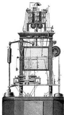
Meteorológiai adatokat rögzítő készülék (1873)
