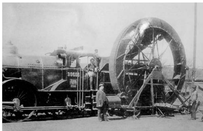
Schilhan-kerek a kanizsai állomáson
